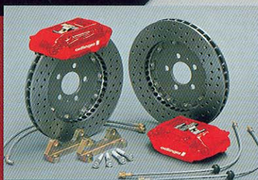
Sportbremsanlage für Vorderachse High performance front brake kit Vierkolben-Festsattelbremse mit 322 / 371 mm-Scheiben four pot-fixed caliper disc brakes 322 / 371 mm discs
